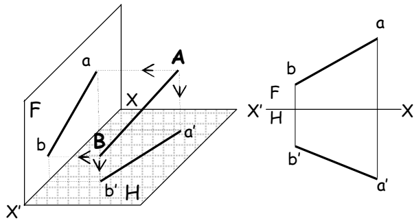
Fig. 5 Projections orthogonales et épure d'une droite quelconque
