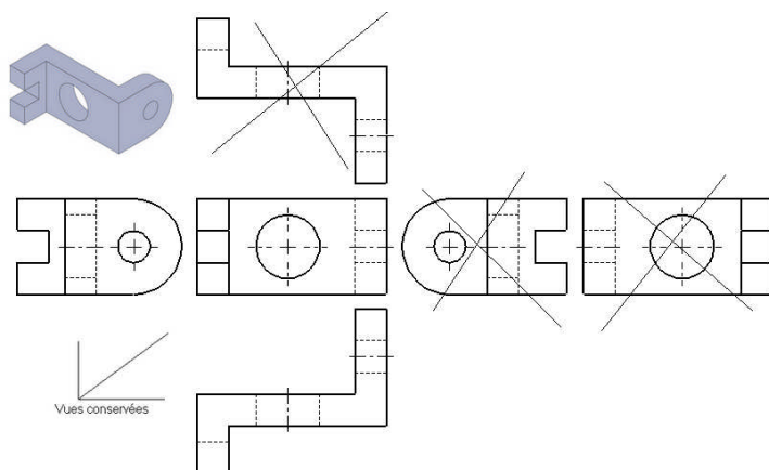
Exemple où deux vues ou une seule vue suffisent
