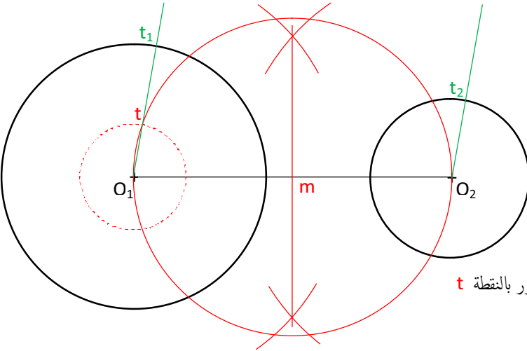
شكل 2 يوضح انجاز دائرة الفرق وتنصيف المسافة بين مركزي الدائرتين ورسم دائرة المنتصف وانجاز
