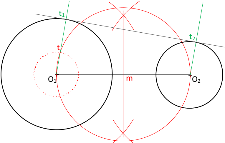
شكل 3 يوضح انجاز المماس الذي يمر بالنقطتين t_1, t_2 دون وجود تقاطع مع الدائرتين أو أي فجوة
